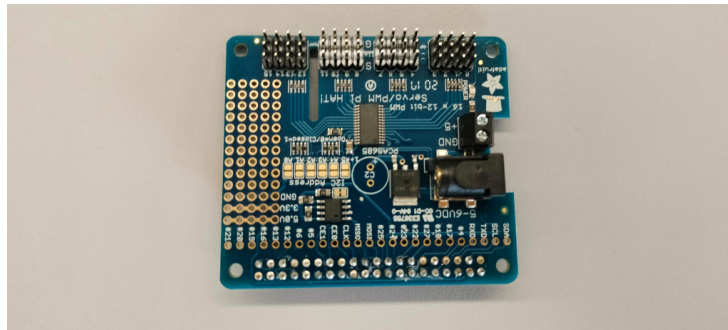
Kit Servo HAT a 16 Canaux pour Raspberry Pi - Kubi
